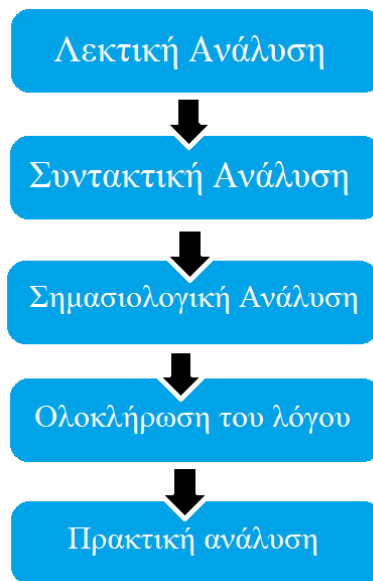
Εικόνα 3-1 Στάδια NLP
