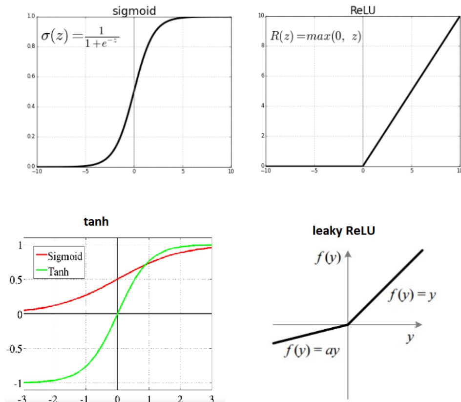
Εικόνα 2-12 Συναρτήσεις ενεργοποίησης
