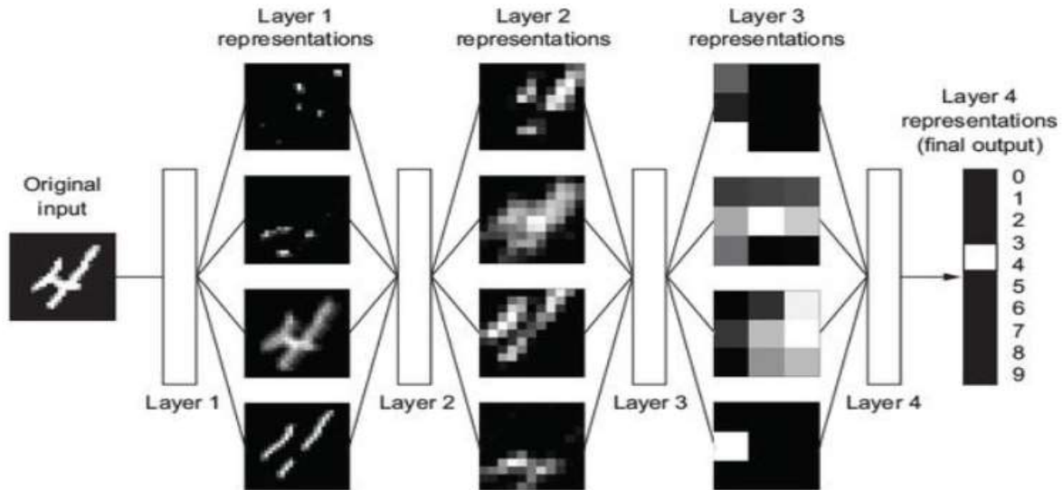
Εικόνα 7: Τα στρώματα αναπαράστασεων ενός μοντέλου βαθιάς μάθησης για την ταξινόμηση ψηφίου [7]
