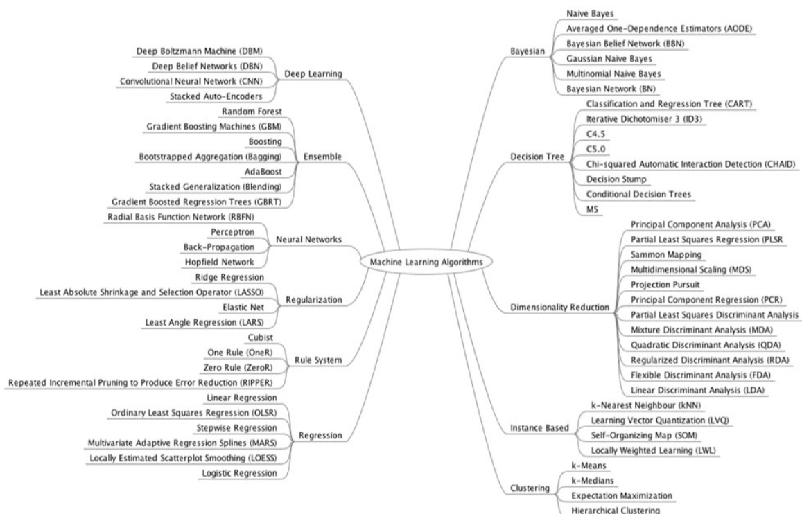
Εικόνα 4: Ταξινόμηση αλγορίθμων μηχανικής μάθησης [95]
