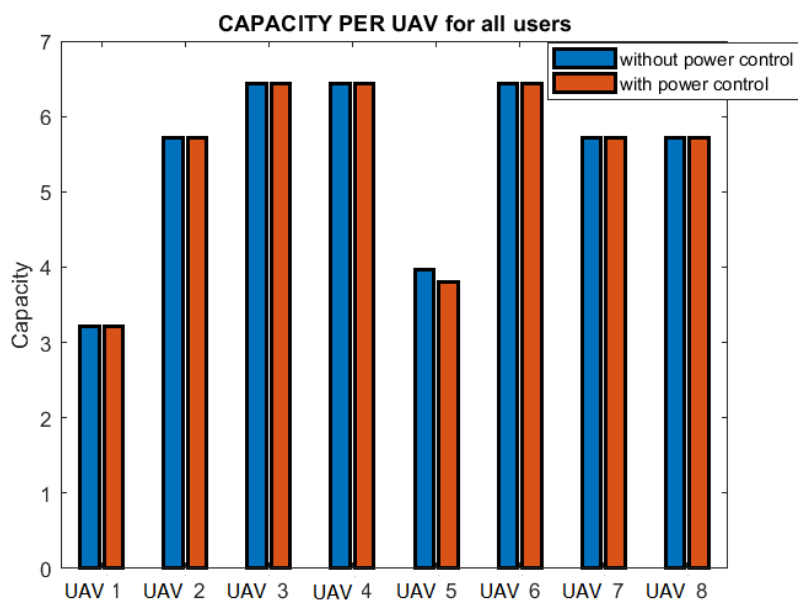
Σχήμα 39: Χωρητικότητα καναλιού για κάθε UAV
