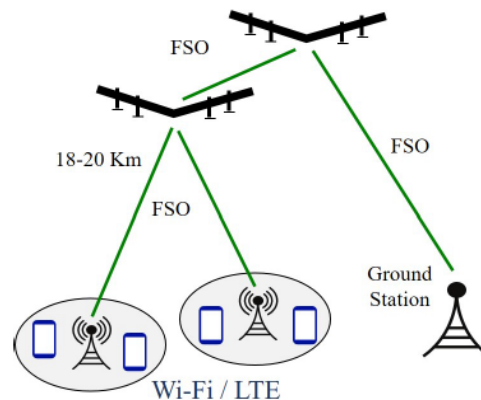
Σχήμα 6: Παρουσίαση της αρχιτεκτονικής Facebook Aquila [29]
