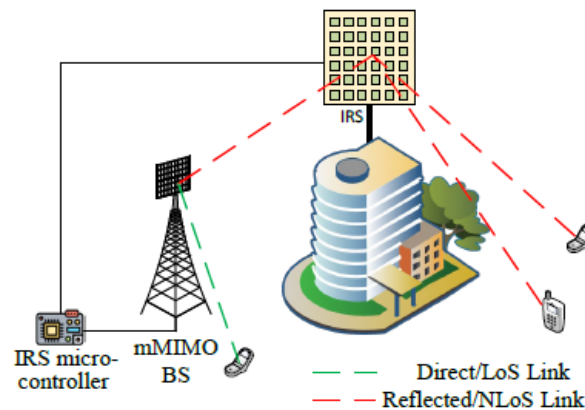
Σχήμα 2: Ύπαρξη έξυπνης αναδιαμορφώσιμης επιφάνειας σε τηλεπικοινωνιακό σύστημα [14]
