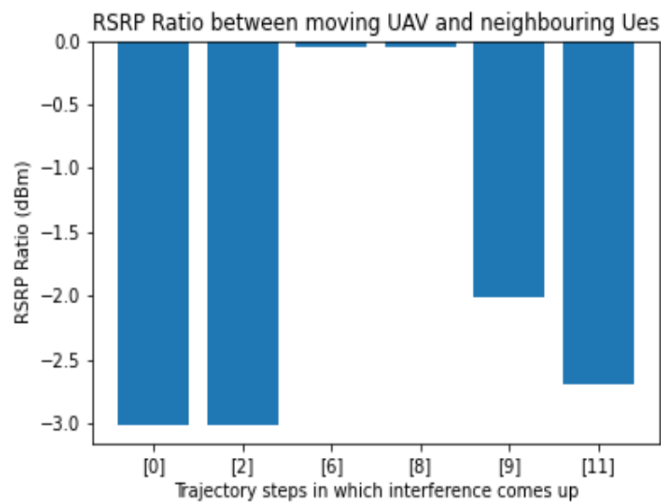
Σχήμα 25: Απεικόνιση του RSRP ratio για τα states που αντιμετωπίζουν παρεμβολή
