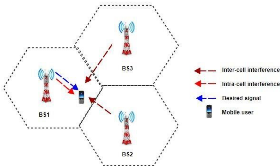
Σχήμα 14: Παρεμβολές Inter-cell και Intra-cell [79]
