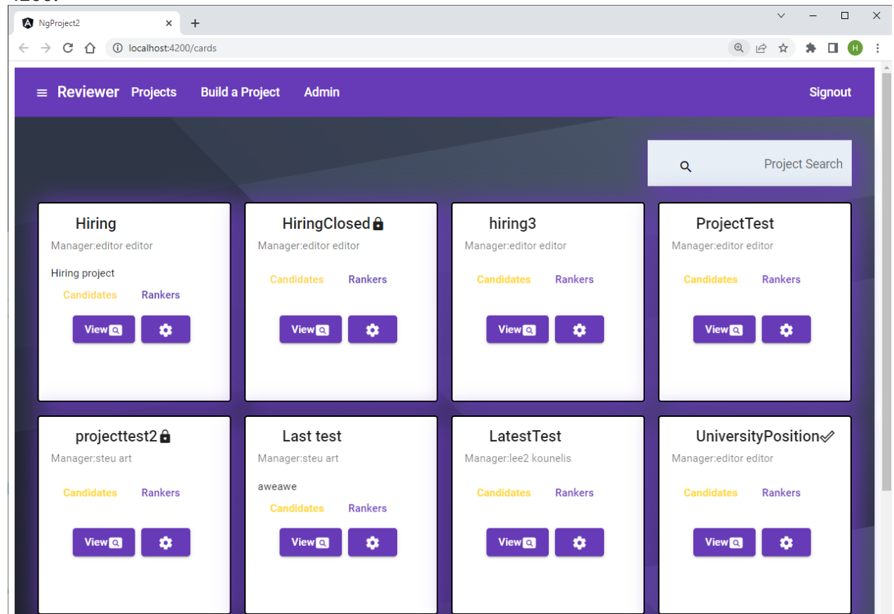
Εικόνα 61 – Εκτέλεση εφαρμογής
