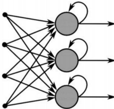
Figure 3.14: Επαναλαμβανόμενο Νευρωνικό Δίκτυο “Τροποποιήθηκε από την πηγή: ΧΑΤΖΗΧΡΙΣΤΑΚΗΣ Φ, 2018”
