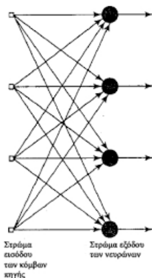
Figure 3.10: Δίκτυα Εμπρός Τροφοδότησης Ενός Επιπέδου “Τροποποιήθηκε από την πηγή: ΧΑΤΖΗΧΡΙΣΤΑΚΗΣ Φ, 2018”
