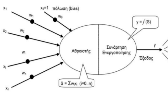
Figure 3.1: Μοντέλο Τεχνητού Νευρώνα “Πηγή: NEURAL NETWORKS AND LEARNING MACHINES”
