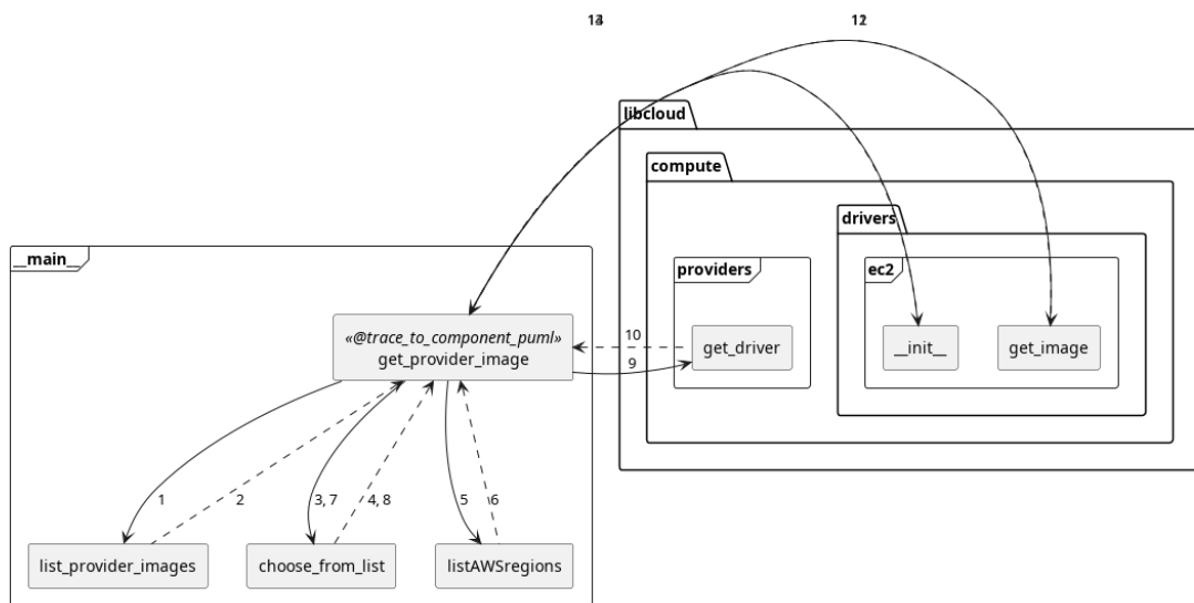
Σχήμα 4.13: Διάγραμμα συστατικών για την Εντολή 2
