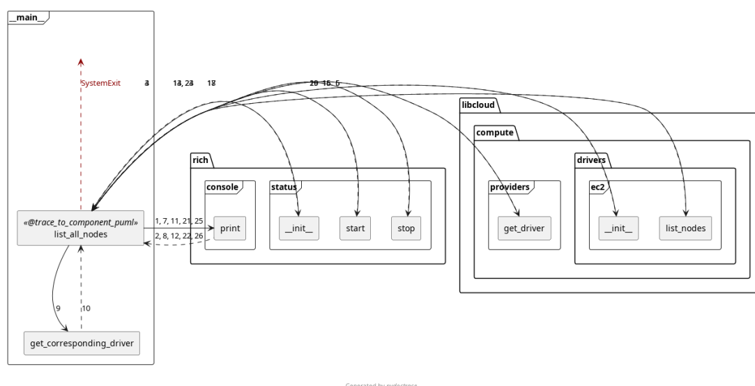
Σχήμα 4.14: Διάγραμμα συστατικών για την Εντολή 3
