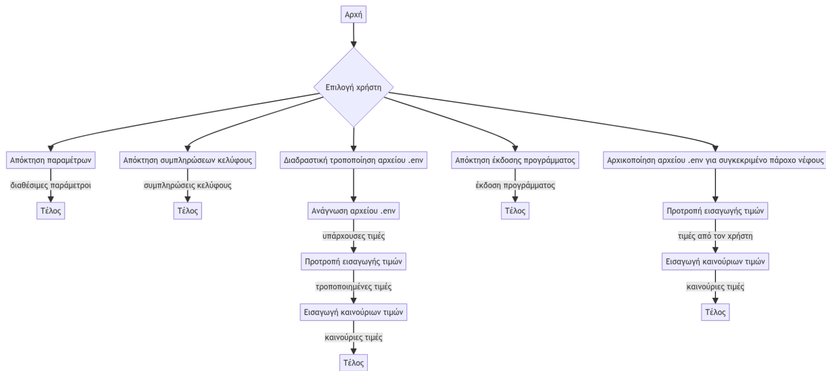
Σχήμα 4.3: Διάγραμμα ροής - Απλές λειτουργίες
