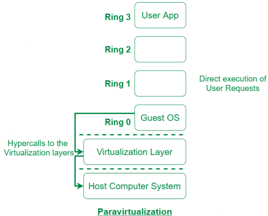
Σχήμα 2.13: Παρα-εικονικοποίηση [45]
