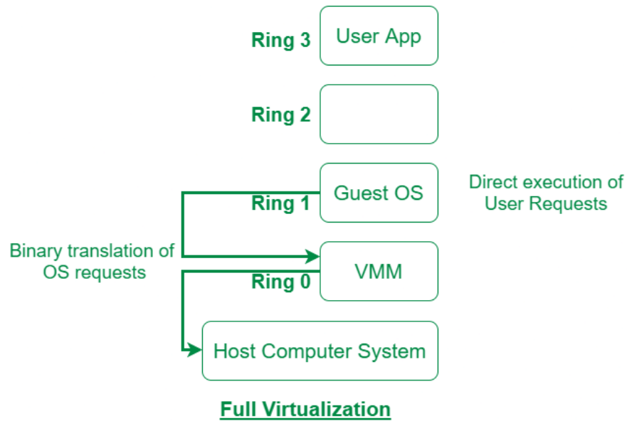
Σχήμα 2.12: Πλήρης εικονικοποίηση [45]
