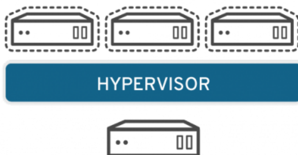
Σχήμα 2.3: Εικονικοποίηση Διακομιστών [20]
