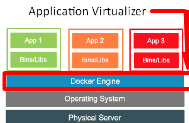
Σχήμα 2.8: Εικονικοποίηση Εφαρμογών [31]
