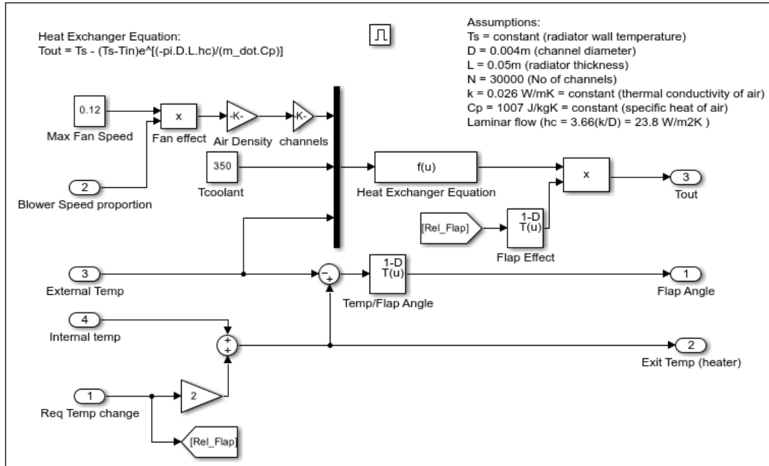
Εικόνα 4.3: Heater Control
