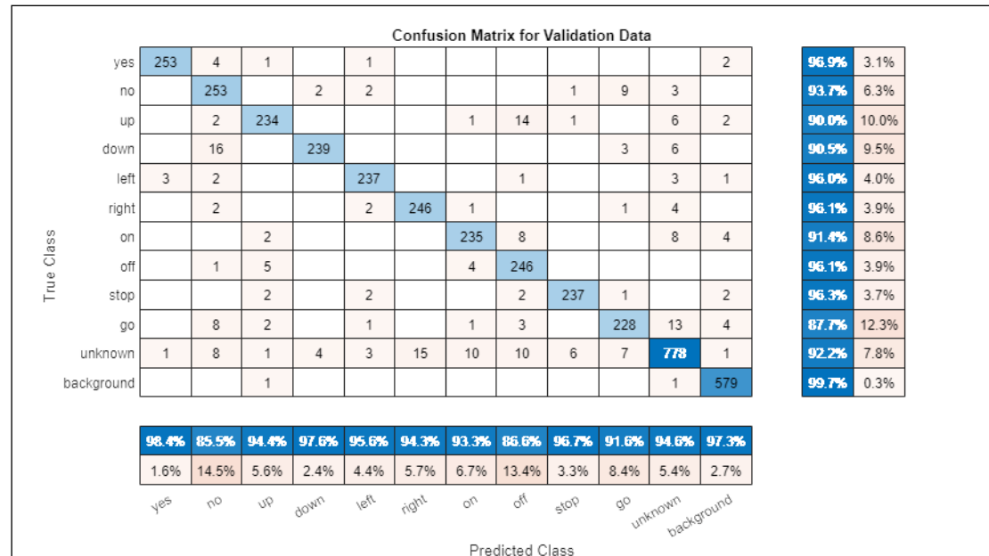
Εικόνα 4.12: Confusion Matrix
