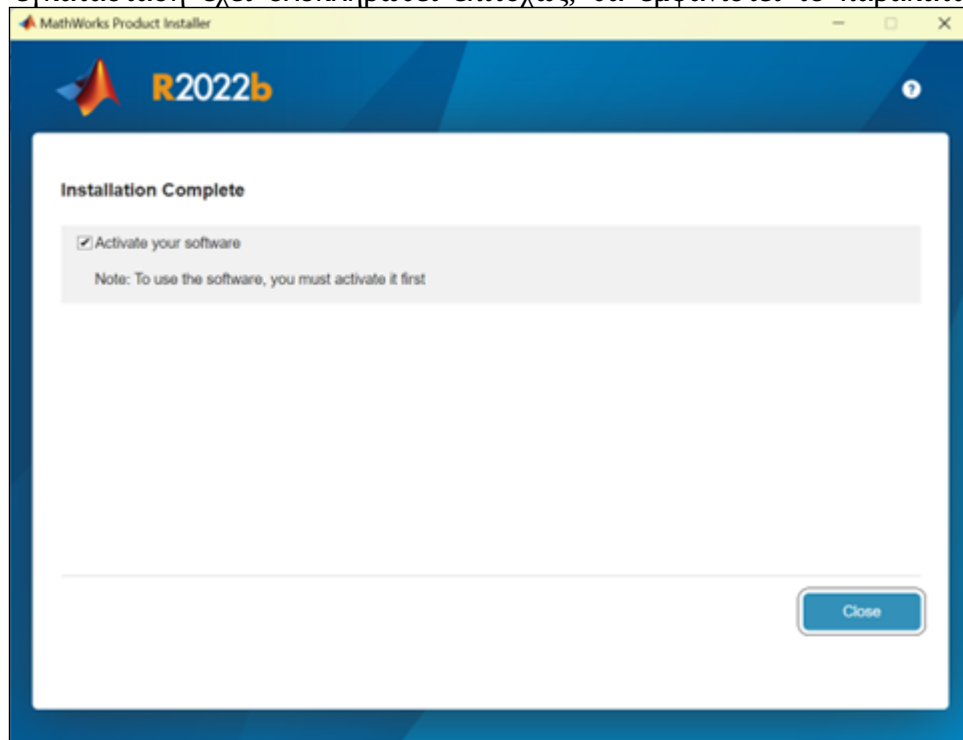
Εικόνα 3.13: Ολοκλήρωση Εγκατάστασης
