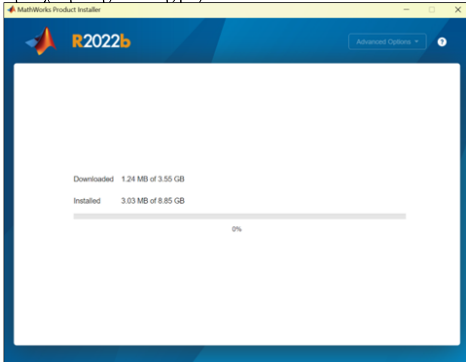
Εικόνα 3.12: Εγκατάσταση
