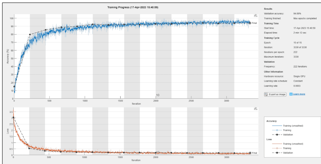
Εικόνα 4.11: Πρόοδος εκπαίδευσης
