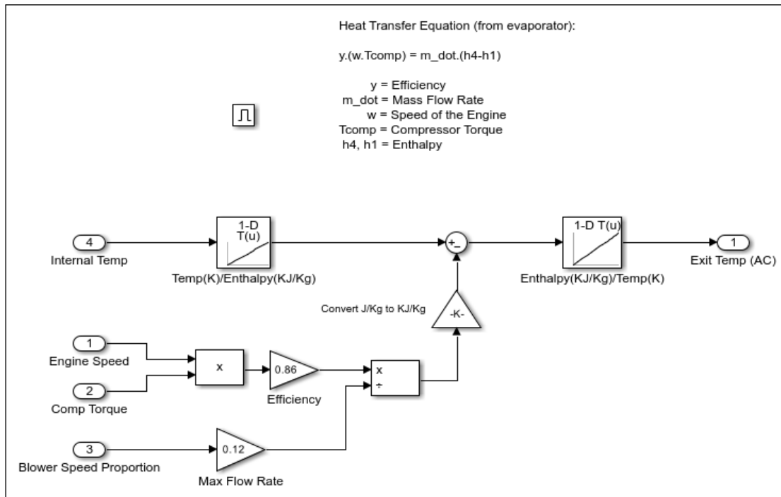
Εικόνα 4.4: A/C control
