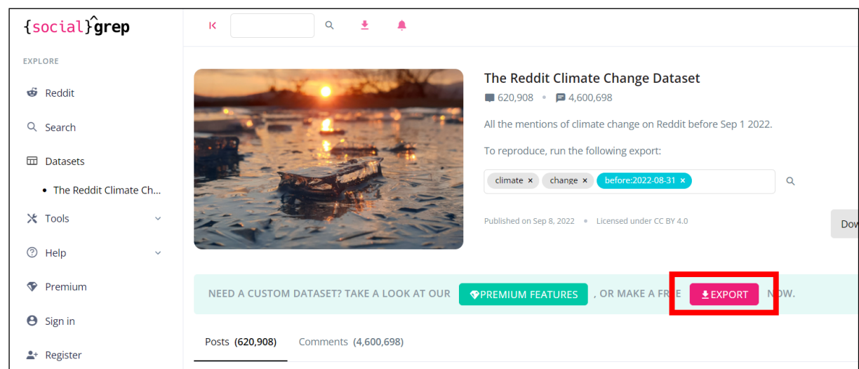
Εικόνα 5.1: Reddit Dataset
