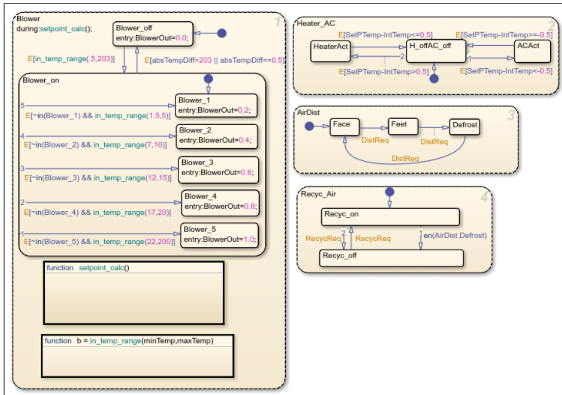
Εικόνα 4.2: Stateflow Diagram
