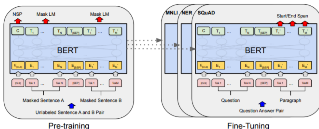
Εικόνα 11: Απεικόνιση της αρχιτεκτονικής του μοντέλου BERT
